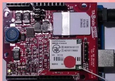
IEM製品版 3Gシールド Ver.1.0
