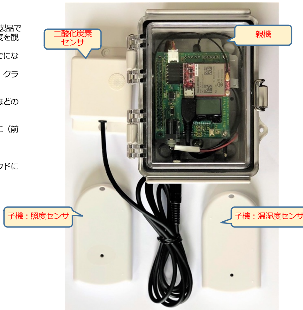
農業用IoT監視デバイス
